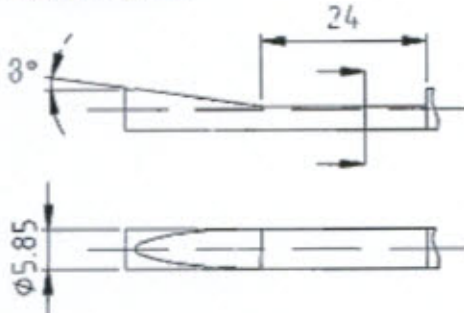
3 Druckfeder
