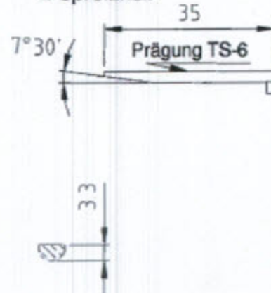
2 Spreizkeil
